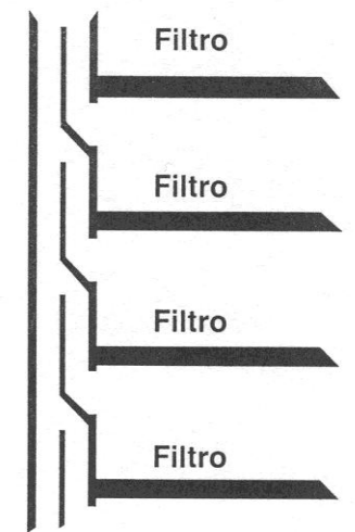
FILTRI A PROVA DI FUMO porte con a.c. e strutture R.E.I. \geq 60
