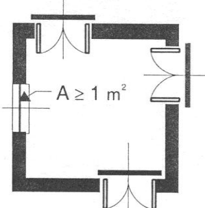
FILTRI A PROVA DI FUMO porte con a.c. e strutture R.E.I. \geq 60
